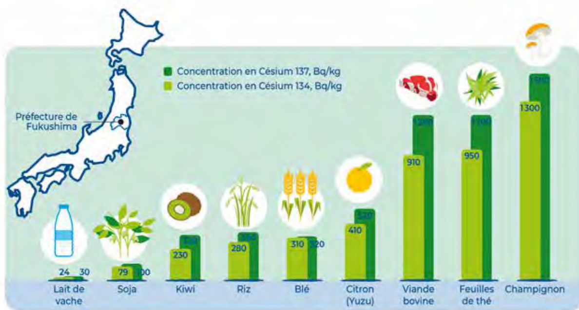
Figure 17. Niveaux d'activité massique en césium 134 et 137 mesurés dans quelques aliments la première année après l'accident de Fukushima (source ASNR)
