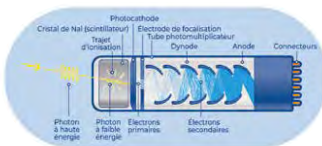
Figure 5. Principe des détecteurs à cristal de NaI
