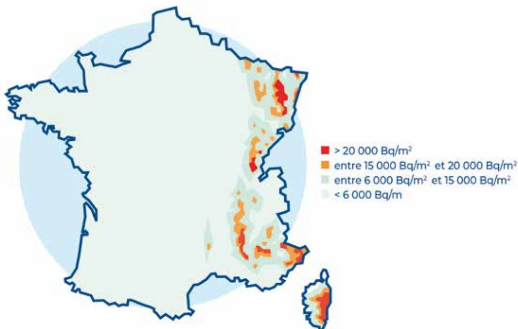
Figure 15. Carte des activités surfaciques actuelles du césium 137 sur les sols de la métropole française (Bq/m²) liées à la rémanence des retombées des essais d'armes nucléaires et de l'accident de Tchernobyl (© IRSN 2019)
