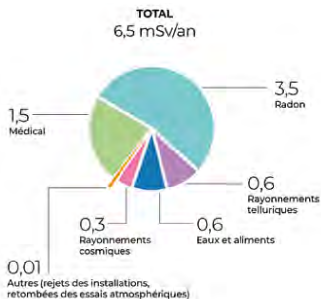
Figure 13. Exposition moyenne aux rayonnements ionisants de la population en France (mSv/an) (Source IRSN 2021)
