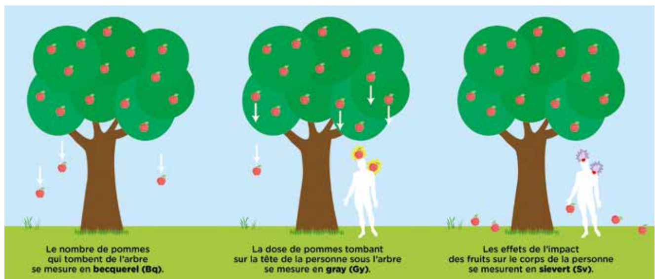
Figure 1. Une représentation de ces trois grandeurs en image. Si la source radioactive est comparée à un pommier...
