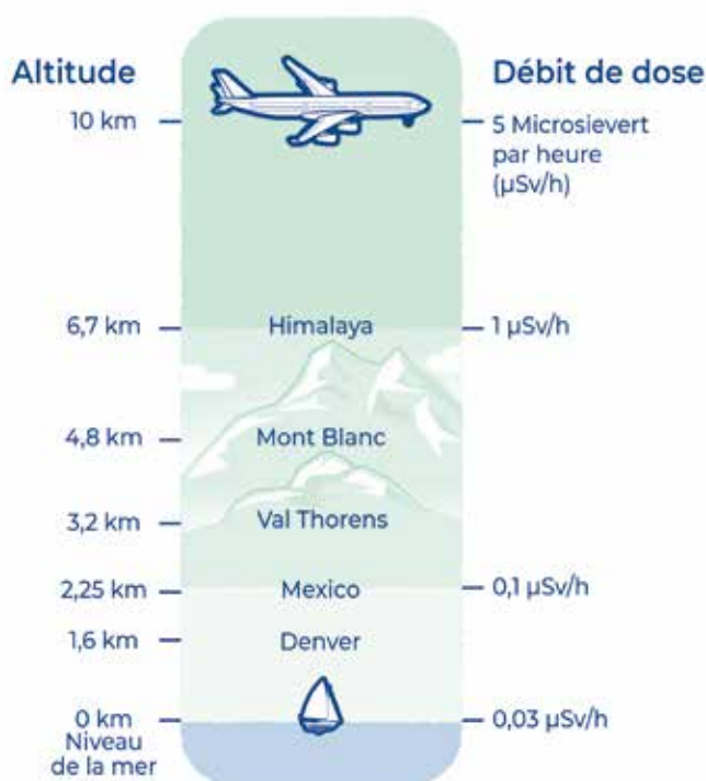
Figure 12. Évolution du débit de dose ambiant avec l'altitude (μSv/h)
