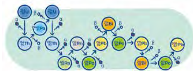
Figure 3. Exemple de la chaîne de désintégration de l'uranium 238.
